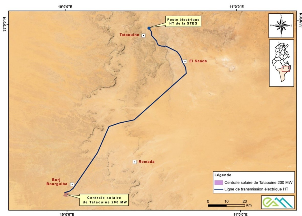
Carte de localisation du projet : centrale photovoltaïque et ligne de raccordement
